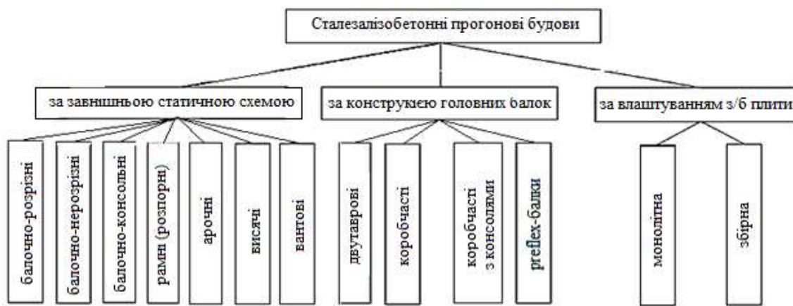
Рис. 1. Різноманітність СТЗБ прогонових будов
