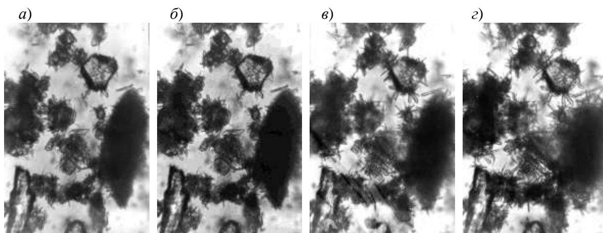
Рис. 2. Мікрофотознімки суміші півгідрату сульфату кальцію і меленого доменного гранульованого шлаку через 5 (а), 10 (б), 15 (в) і 20 хвилин (г) після замішування водою. Знімки отримані А.А. Плугінін та О.Г. Ольгінським у 1993 р. за допомогою мікроскопа МБИ-6 ЛОМО
