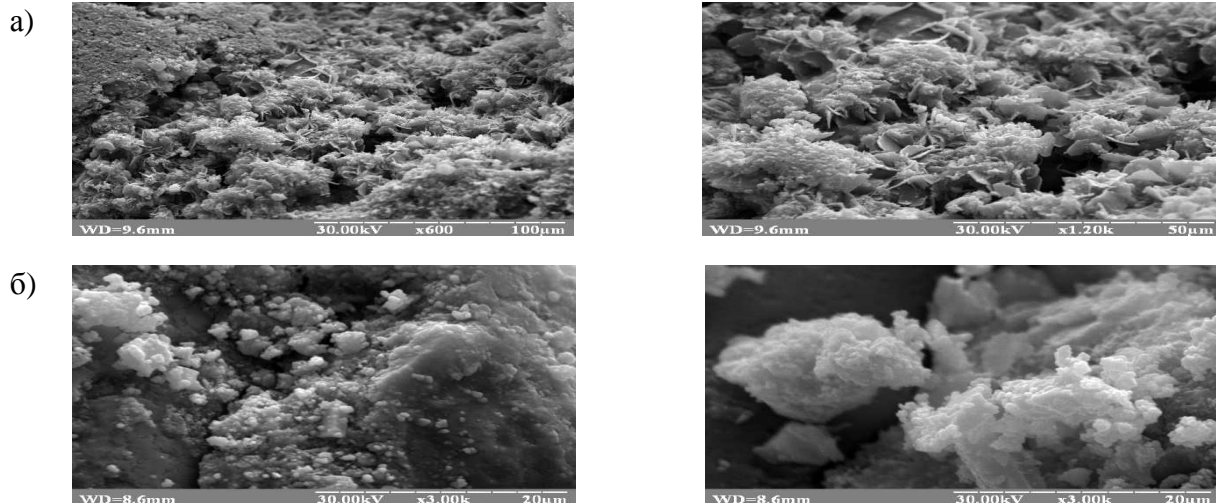
Рис. 2. Фотографії поверхні зламу штучного каменю після 3-х років твердіння, отриманого на основі: а – портландцементу з добавкою доменного гранульованого шлаку та природного цеоліту; б – портландцементу з добавкою доменного гранульованого шлаку, природного цеоліту і солей-електролітів (фото зламу штучного каменю отримані за допомогою електронного мікроскопа РЕММА-102)
