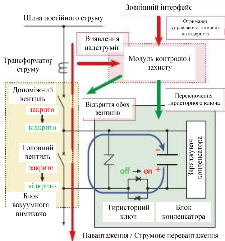
Рис. 9. Принцип вимикання постійного струму за допомогою HSCB
