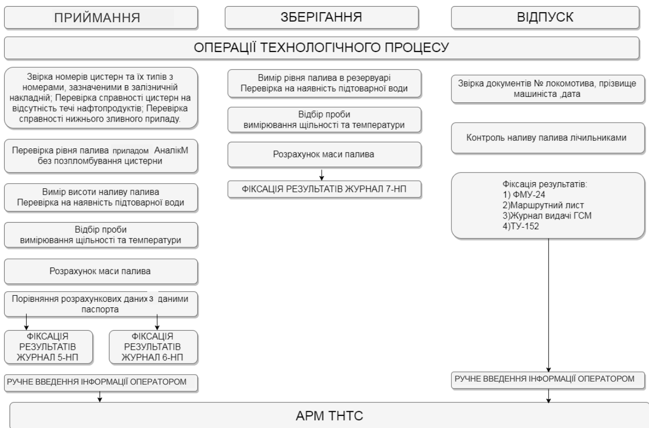
Рис. 1. Технологічний процес використання дизельного пального
