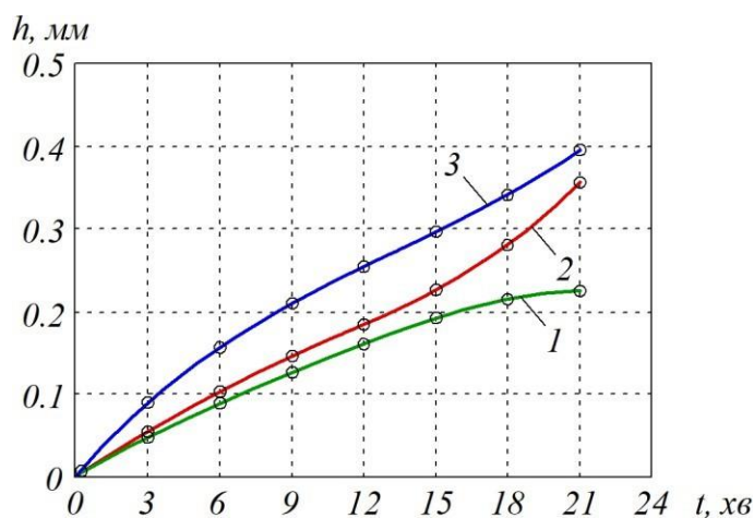
Рис. 2. Залежність зношування по задній поверхні від тривалості обробки сталі ШХ15 (HRC 60...62) пластинами: 1 – з \text{Al}_2\text{O}_3 –50 мас.% WC; 2 – ВОК-71; 3 – ВО-13 (режим різання: v \times s \times t = 200 \text{ м/хв} \times 0,085 \text{ мм/об} \times 0,2 \text{ мм} )
