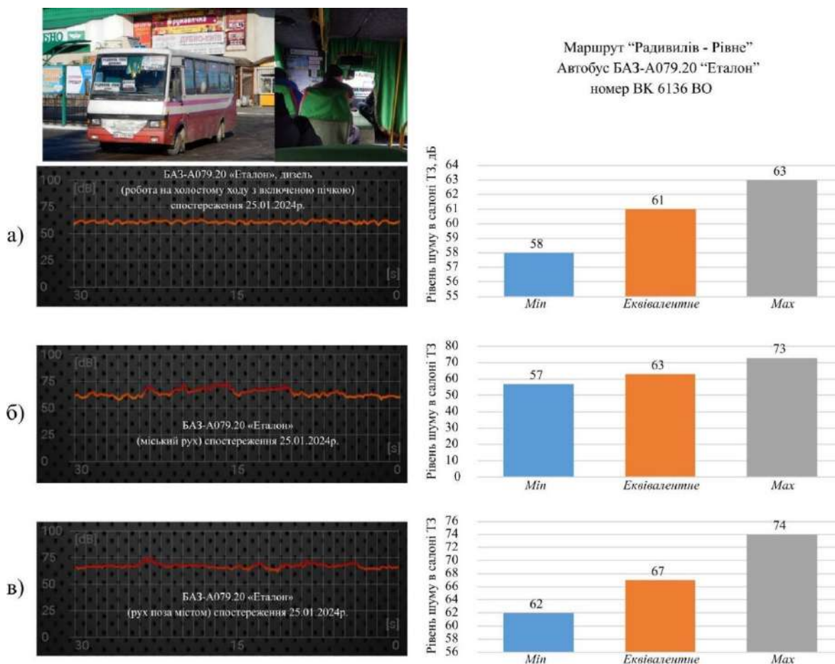
Рис. 6. Шумове навантаження в салоні автобуса за роботи на холостому ходу (а), під час руху в міських (б) і позаміських (в) умовах
