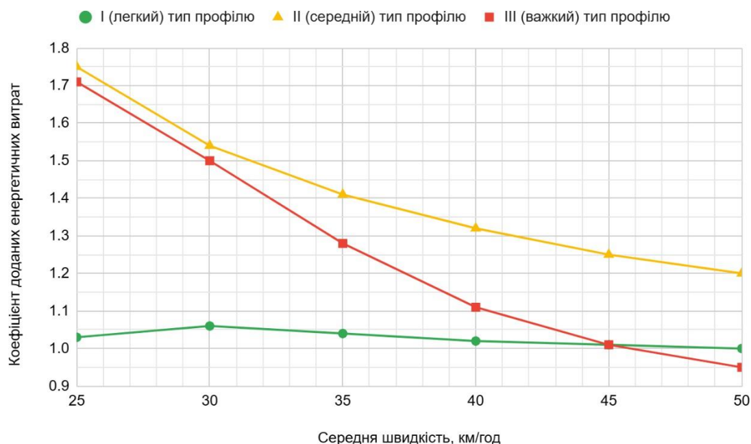
Рис. 6. Графічне подання залежності КДЕВ від середньої швидкості на типових профілях
