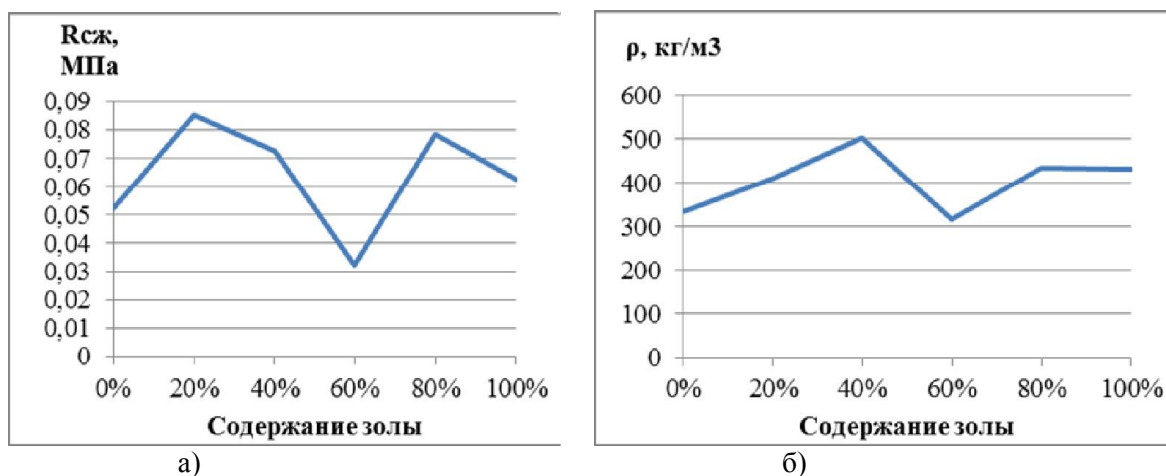
Рис. 2. Влияние содержания золы на: а – прочность при сжатии, МПа; б – плотность, кг/м³
