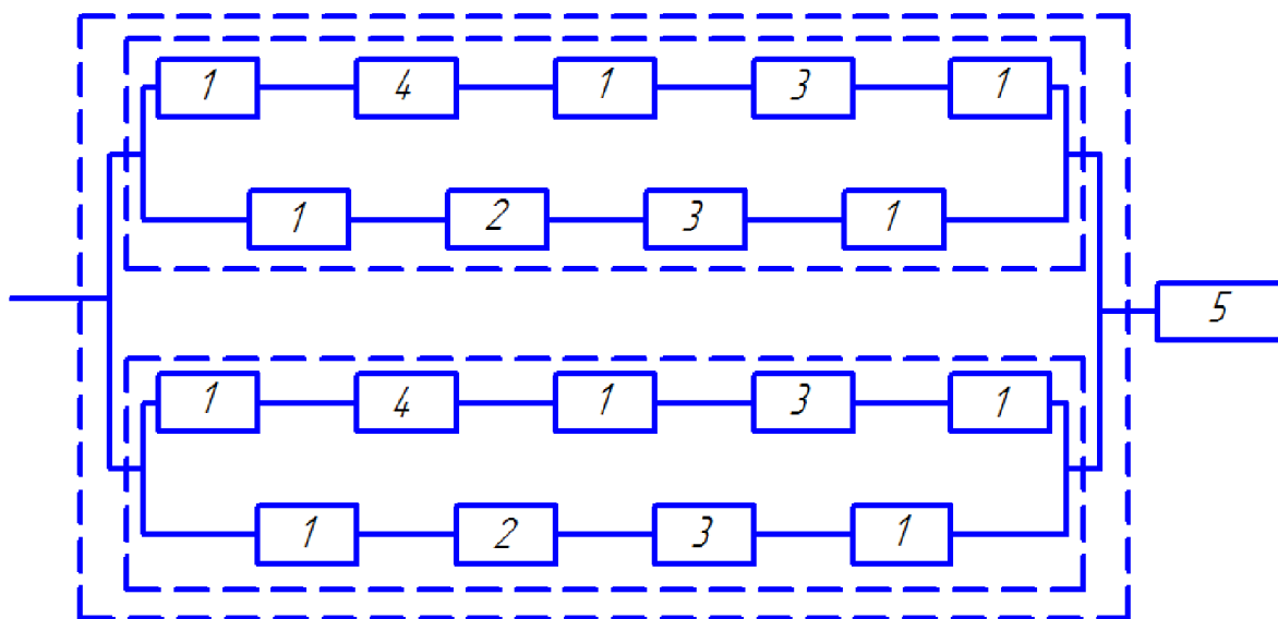
Рис. 2. Структурна схема каретки струмоприймача: 1 – вал; 2 – верхній стрижень каретки; 3 – нижній стрижень каретки; 4 – пружина; 5 – корпус
