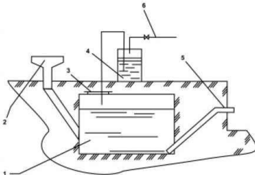
Рис. 1. Схема простейшей БГУ с ручной загрузкой без перемешивания и без подогрева сырья в реакторе: 1 – реактор; 2 – бункер загрузки; 3 – люк для доступа в реактор; 4 – водяной затвор; 5 – выгрузочная труба; 6 – отвод биогаза
