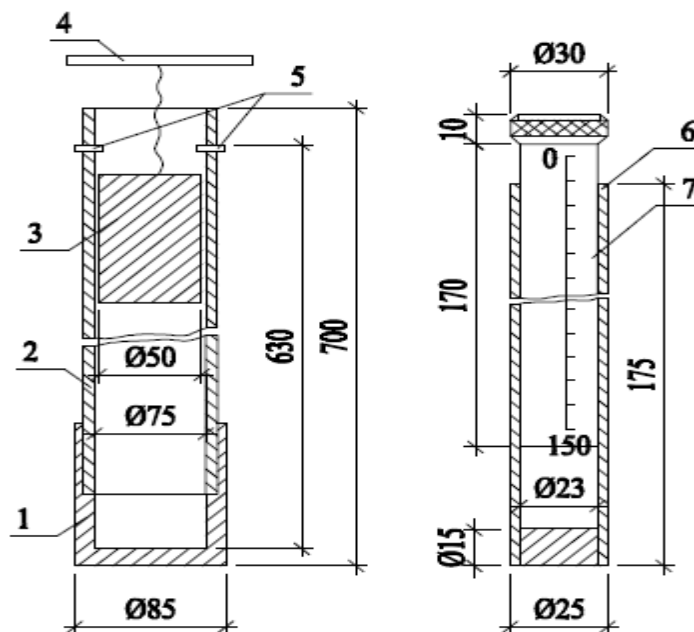
Рис.1. Прибор для определения крепости РОК
