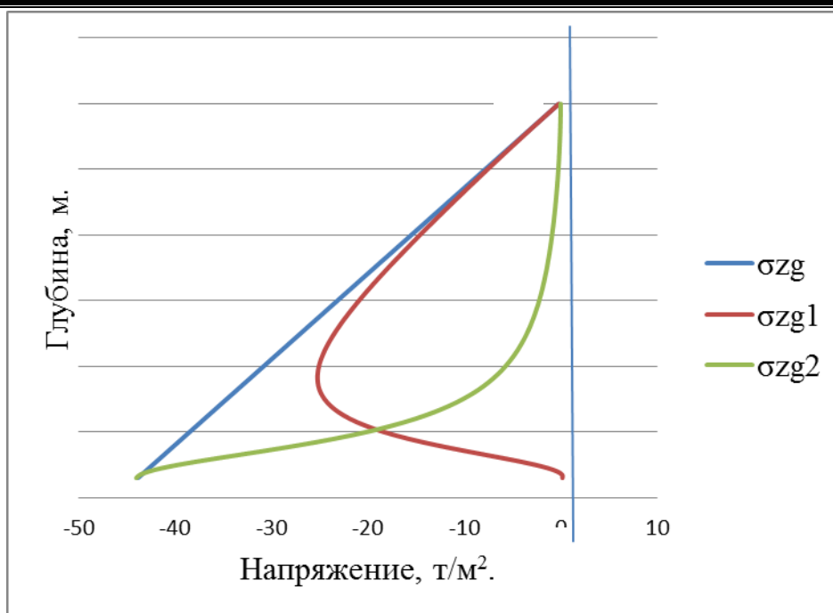
Рис.2. Характер напряженно-деформированного состояния в грунте при выработке в виде прямоугольника.
