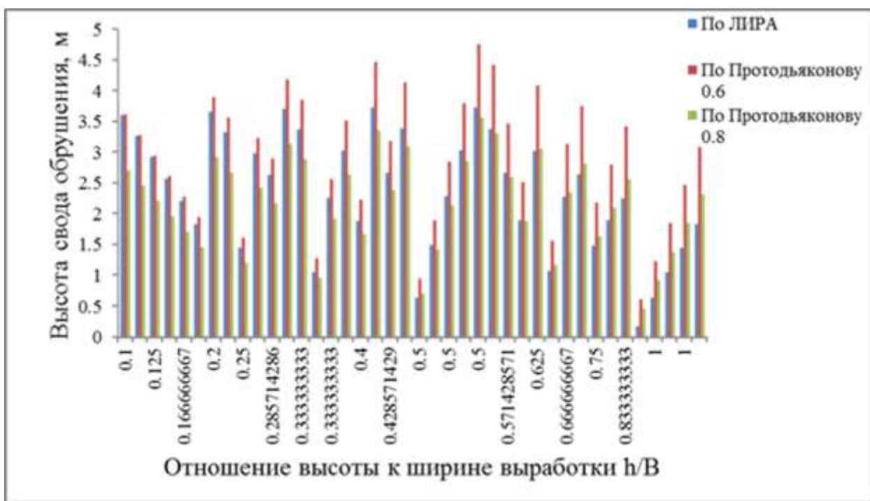
Рис.3. Диаграмма сравнения результатов определения высоты сводаобразования с использованием ПК «ЛИРА» и по методу проф. М.М. Протодяконова.
