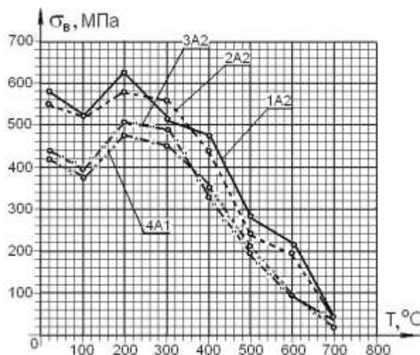
Рис. 3. Зависимости предела прочности арматурной стали от температуры
