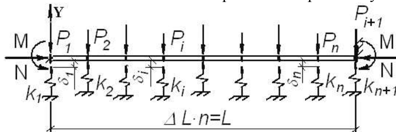
Рис. 1. Расчетная схема изгибаемой системы
