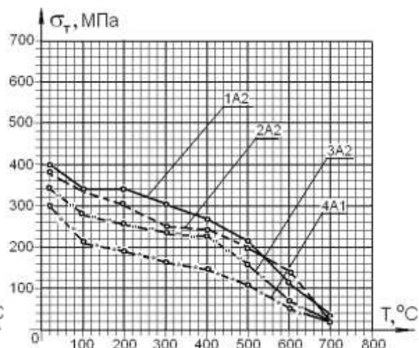
Рис. 4. Зависимость предела текучести арматурной стали от температуры
