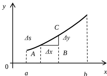
Рис. 1. Длина дуги и геометрической смысл дифференциала дуги и кривизны
