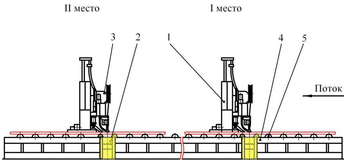
Рис. 3. Универсальный двухместный станок автоматической сварки первой стороны листовых полотнищ:
