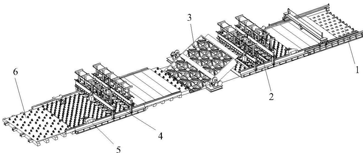
Рис. 1. Линия сборки и сварки листовых полотниц обечаек котлов железнодорожных вагонов-цистерн и контейнеров-цистерн:
