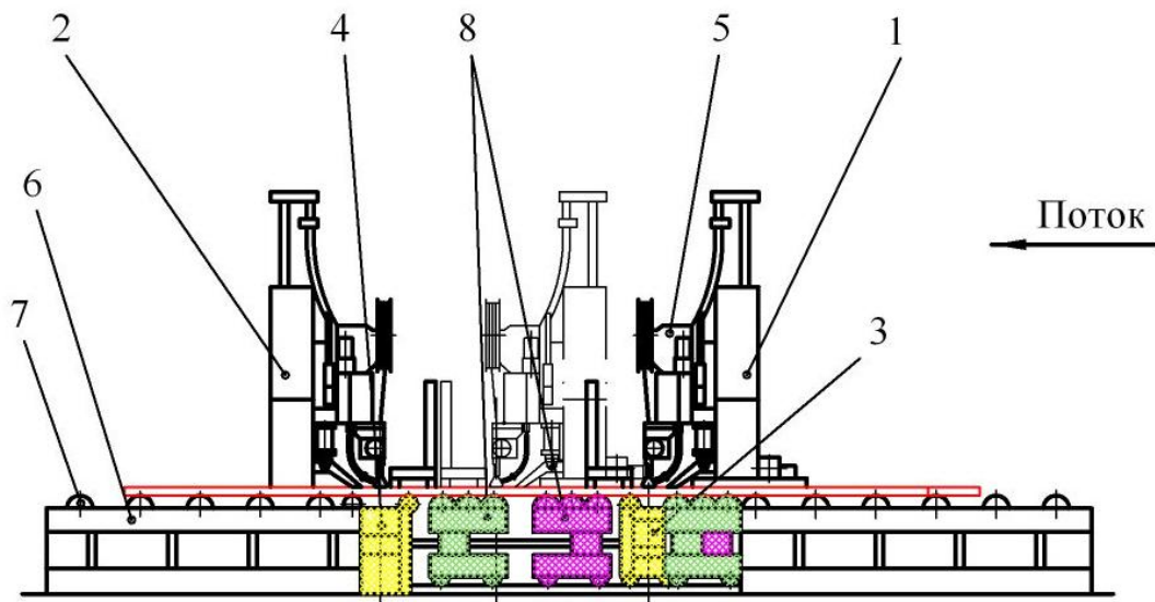
Рис. 2. Универсальный односторонний стан автоматической сварки первой стороны листовых полотнищ:
