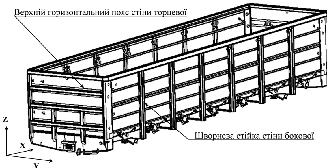
Рис. 2. Загальний вигляд кузова напіввагону
