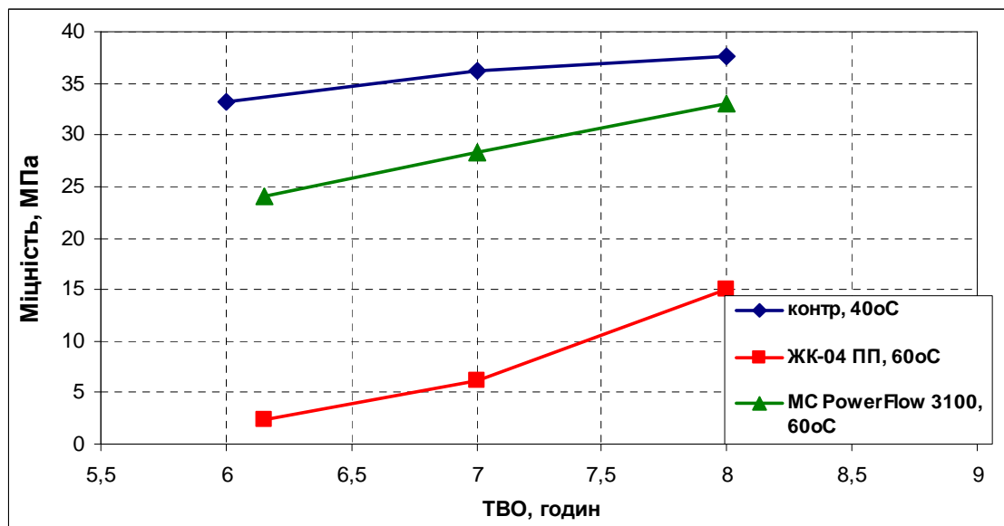
Рис.5. Кінетика набору міцності досліджуваних складів бетону з пластифікаторами та метаксаоліном при T = 60^{\circ}\text{C}
